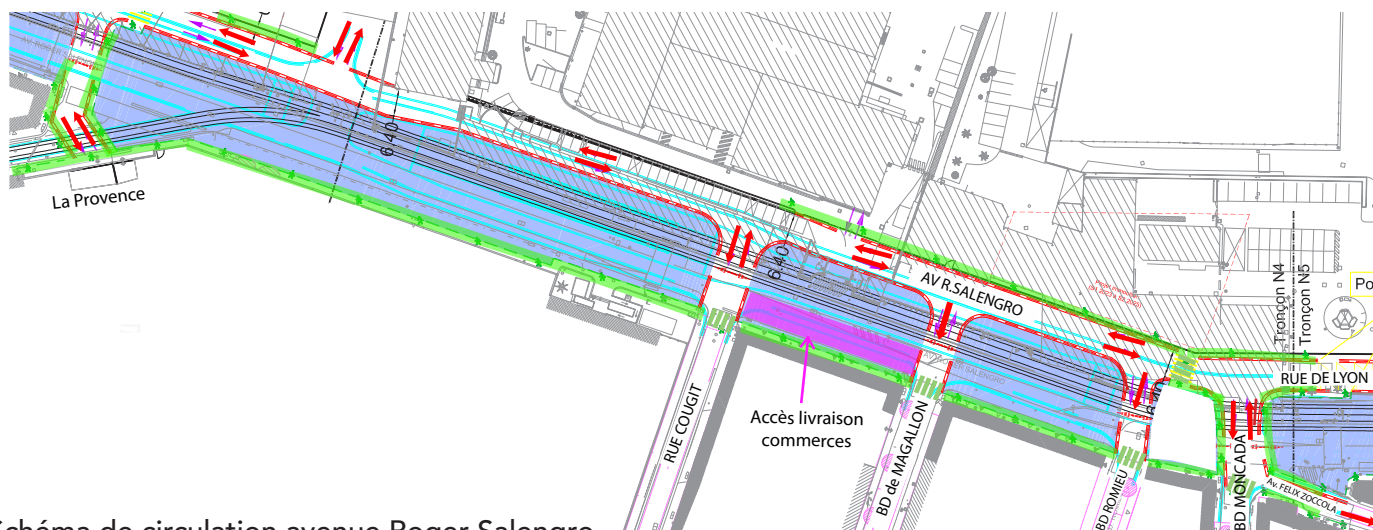
Schéma de circulation avenue Roger Salengro
